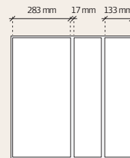
Troldekt® tiles 1 + 2
